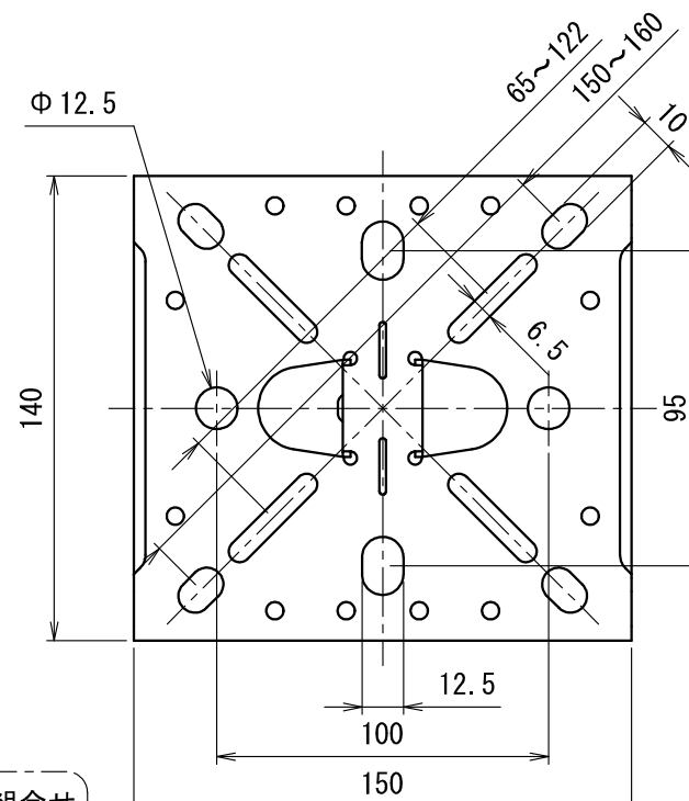
底面図
